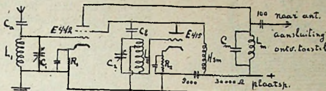
Fig. 2. Voorzetapparaat met wisselstroomlampen. Twee afstemmingen. Goolflengten vanaf 10 m.
