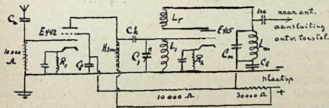
Fig. 1. Voorzetapparaat met wisselstroomlampen. Eénknopsafstemming voor goolfengten vanaf 10 m.
