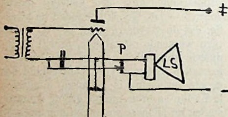
Fig. III. P is een potentiometer van minstens 10 \times luidsprekerweerstand.
