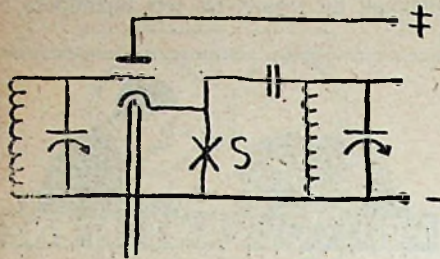
Fig. I. Smoorspoel S zorgt tevens voor neg. roosterspanning.
